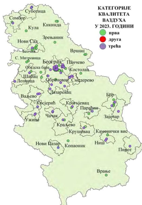
Слика 4.2.4. Категорије квалитета ваздуха у 2023. години на територији Републике Србије
